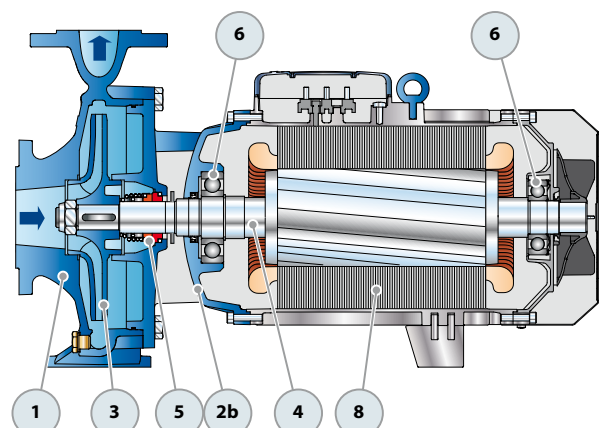
Version triphasée
